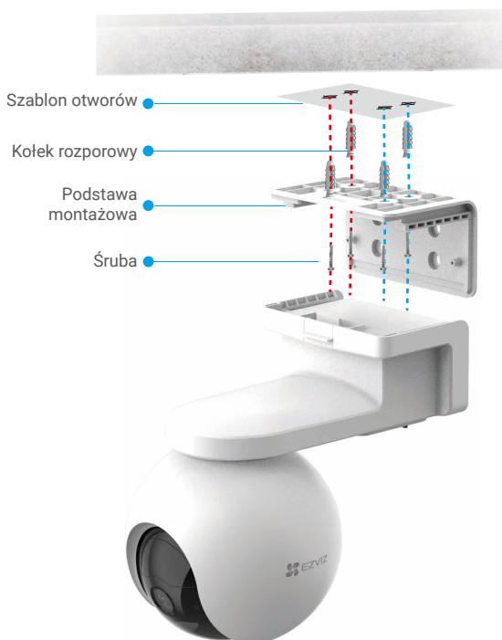
Rys. 1 Montaż sufitowy
